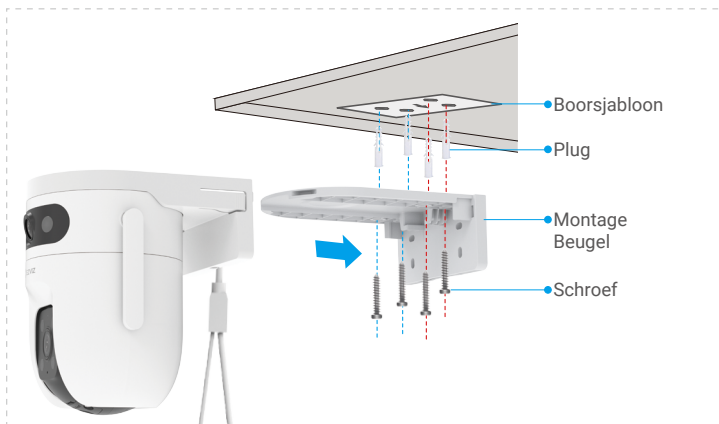
Afb. 1 Plafondmontage
